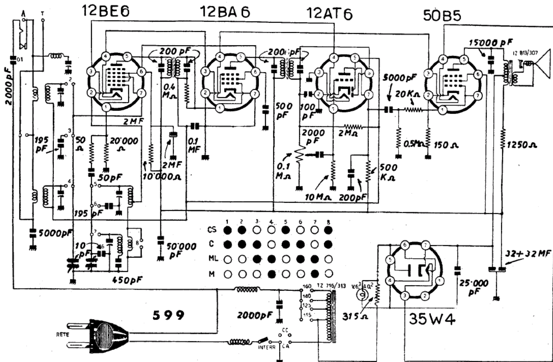
PHONOLA RADIO - Mod. 599 - Medie da 520 a 720 kc e da 680 a 1650 kc; corte da 6 a 8,1 Mc e da 7,9 a 18,1 Mc. MF a 470 kc. Consumo 30 W. Potenza 1,2 W.
